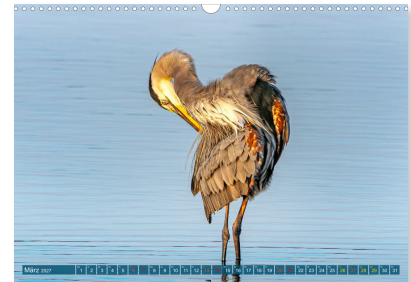
Wunderschöne Verwandte in getrennten Welten 2027
